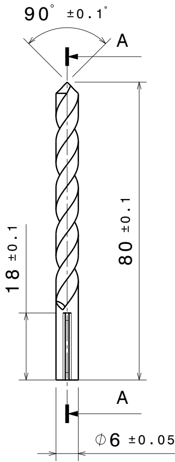
Right view Scale: 1:1
